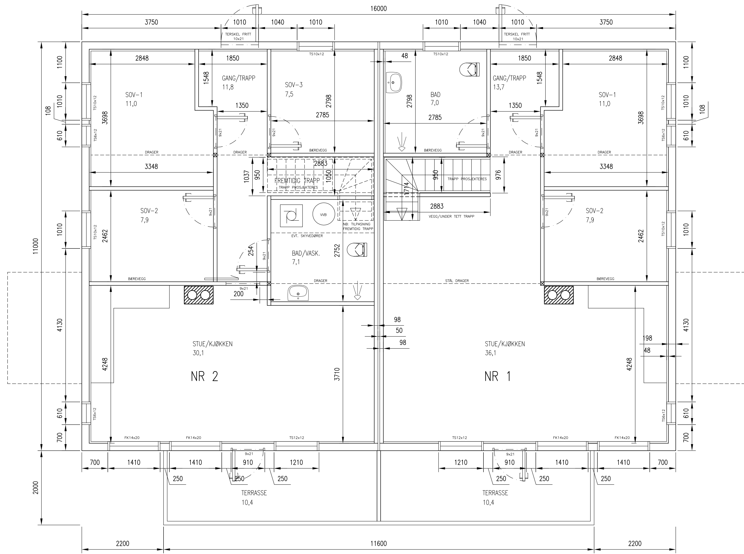
ARBEIDSTEGNING 1. PLAN
