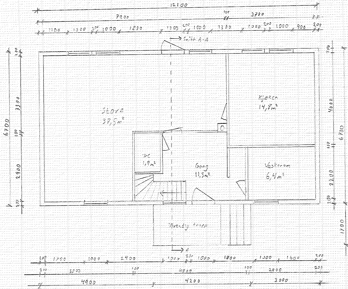
Eksisterende plan 1. etasje
