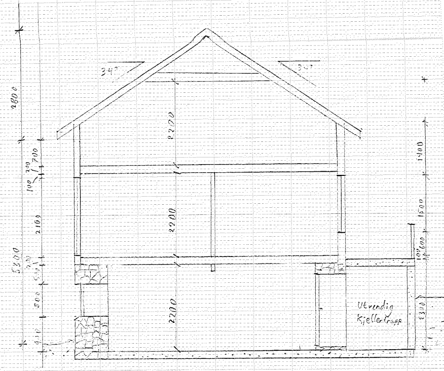
Eksisterende snitt A-A
