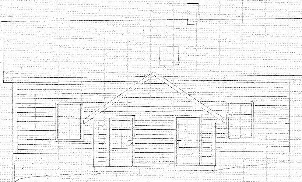
Fasade Nord-aust
