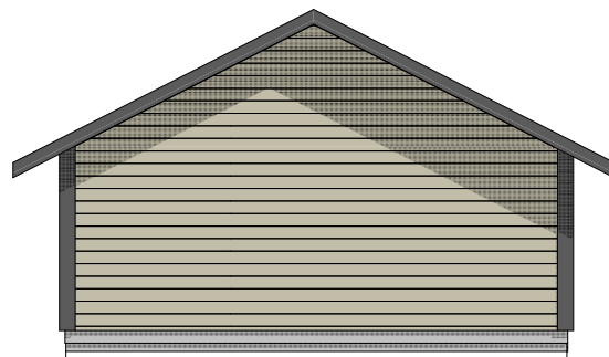
1:100 Fasade Sør-Vest
