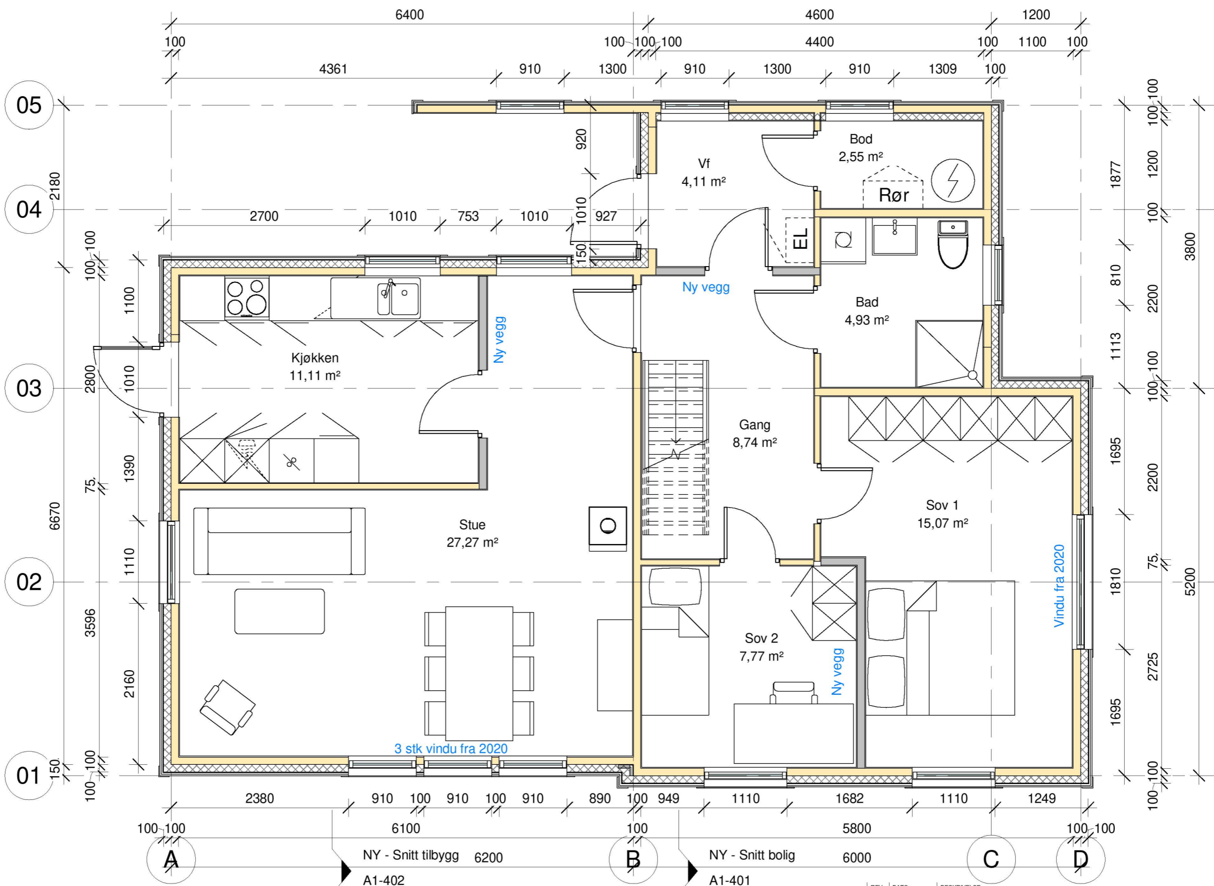
1 NY 1 - hovedplan 1 : 50
