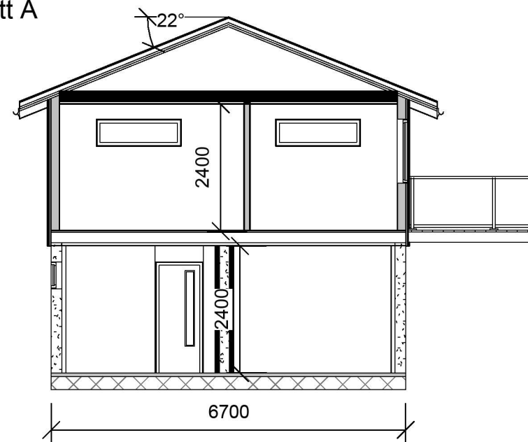
Snitt A
