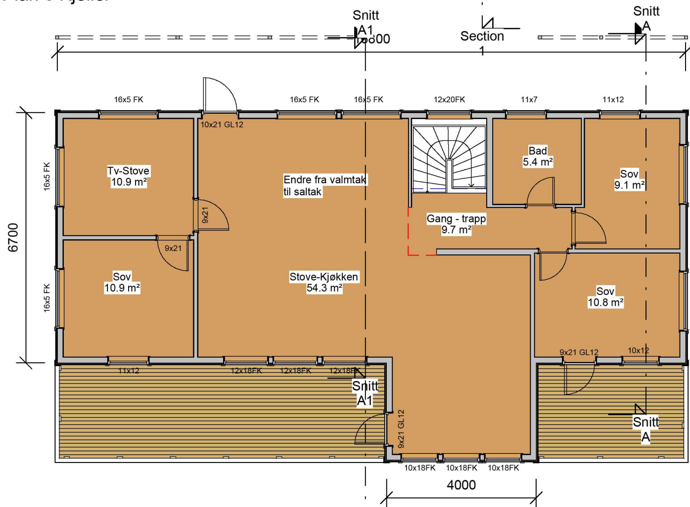
01 Plan 1 Etasje
