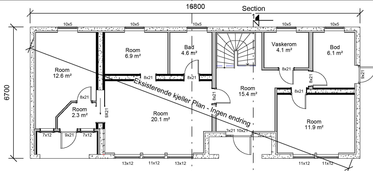
00 Plan 0 Kjeller
