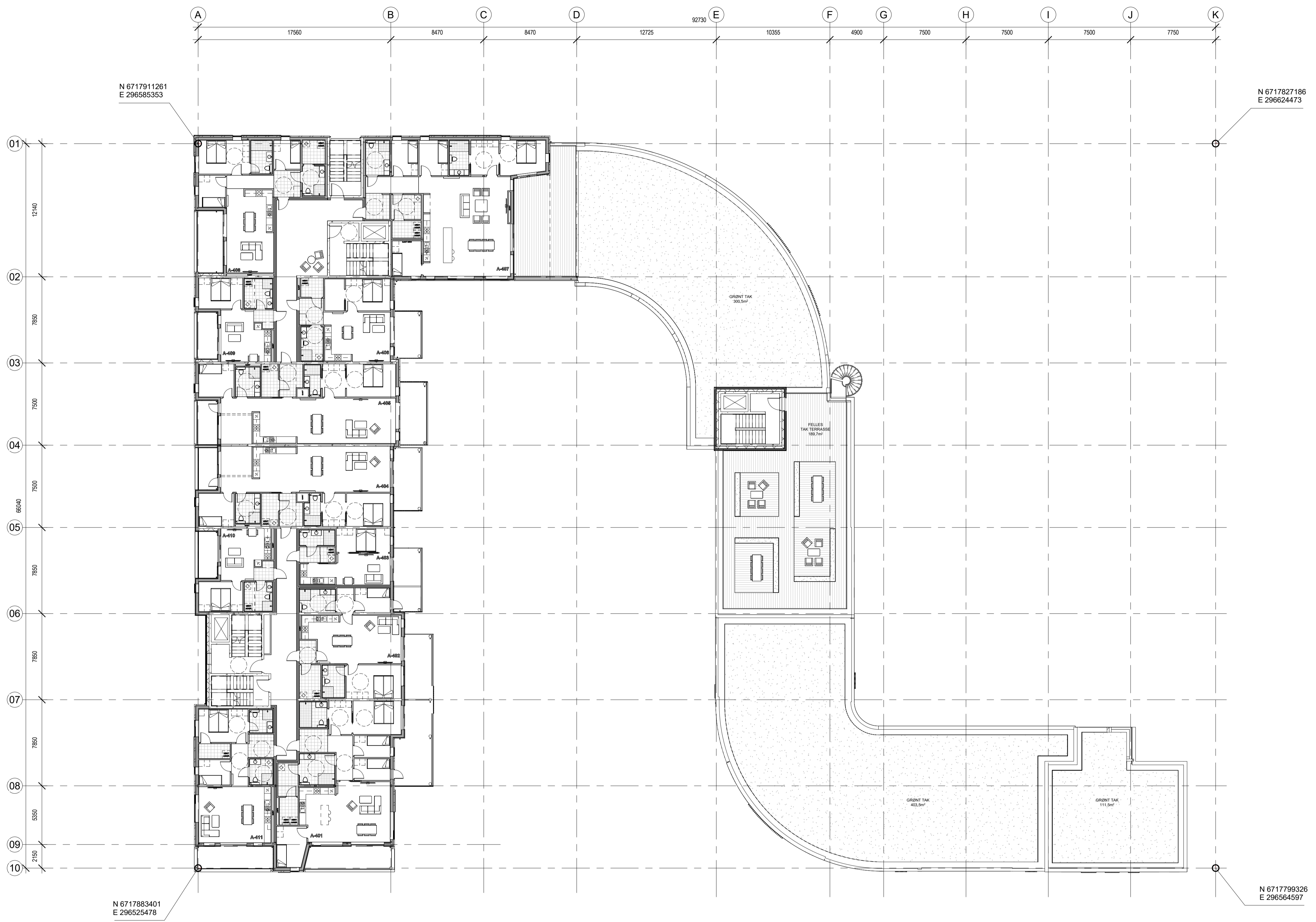
1 4. etasje - 1-200 1 : 200
