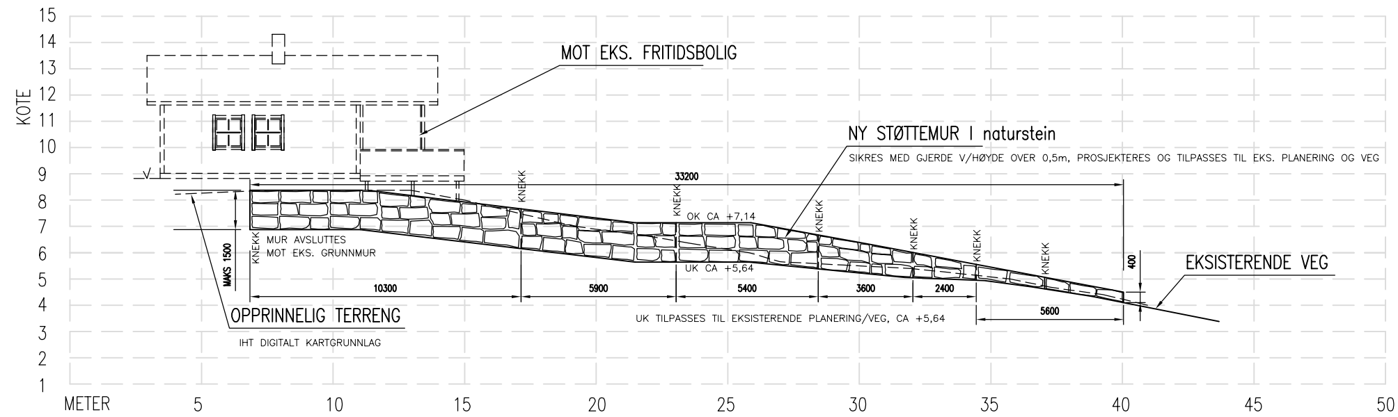
MURPROFIL 2
