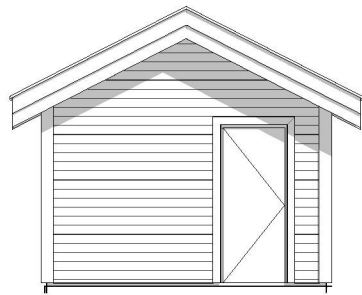
1:100 Fasade Nord
