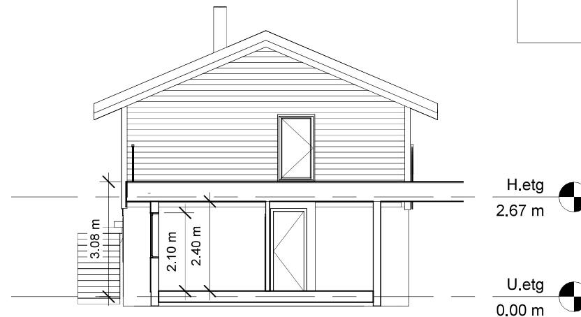
3 snitt 2 1 : 100
