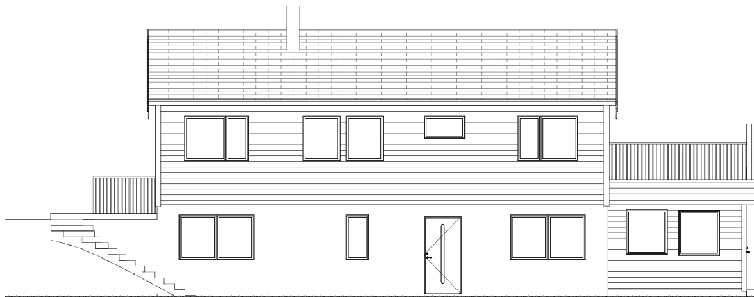
4 Øst 1 : 100
