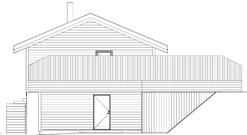
1 Nord 1 : 100
