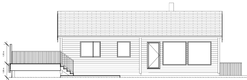
3 Vest 1 : 100
