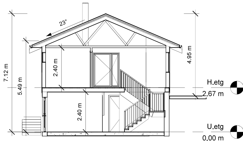
2 snitt 1 1 : 100
