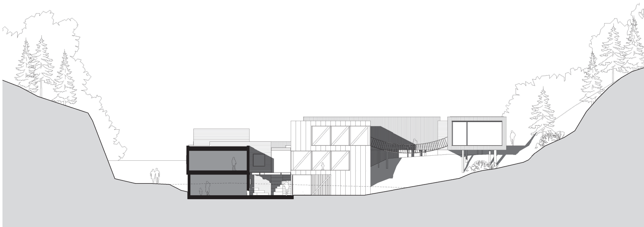
SNITT D-D
