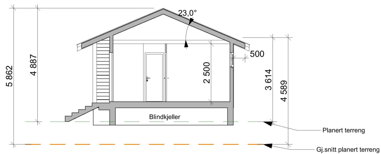
Snitt B
