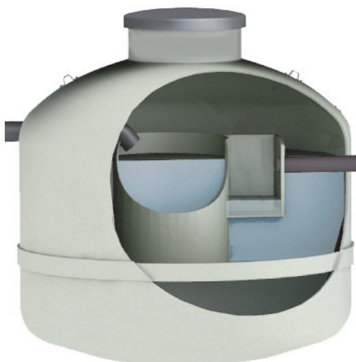
Slamsikringstank ved selvfall
