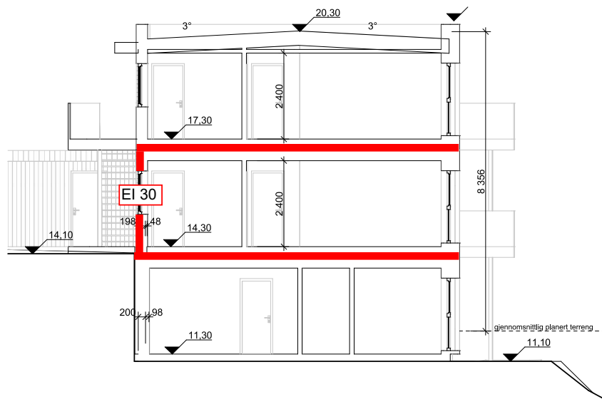
1:100 Snitt H3
