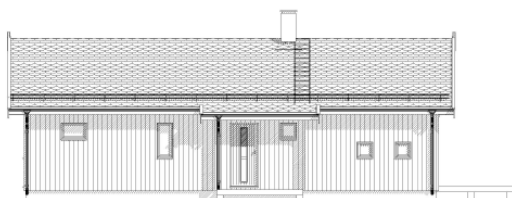
Teikningar av omsøkt hytte på Baløyna
