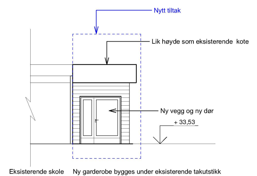
Fasade Nordøst 1 : 100
