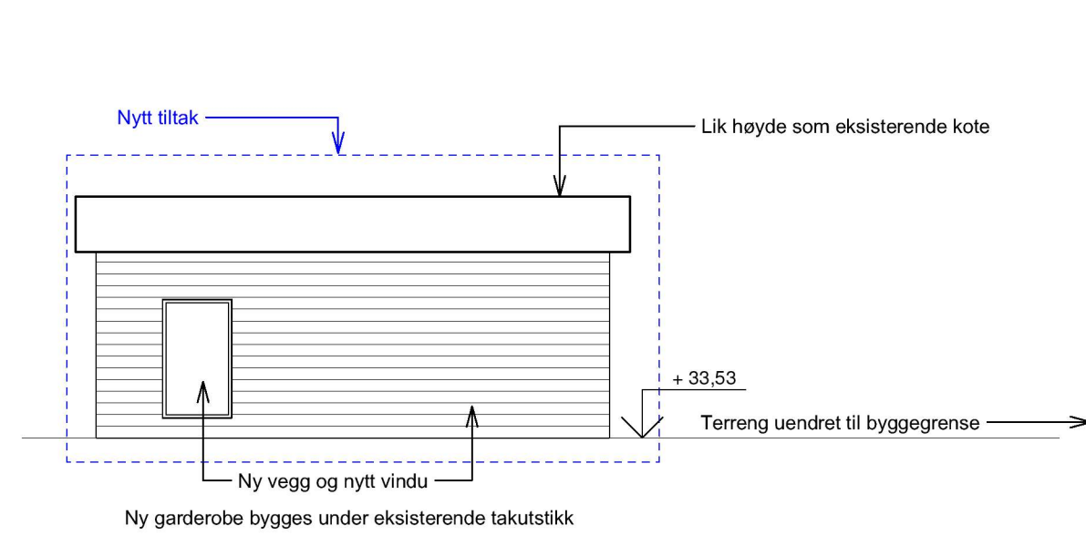
Fasade Nordvest 1 : 100
