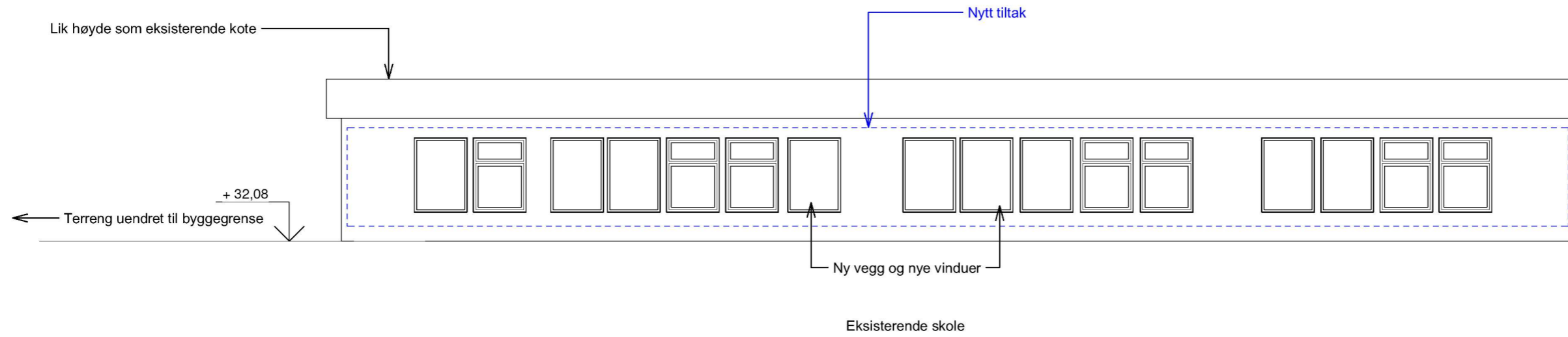
Fasade Nordøst 1. etg 1 : 100
