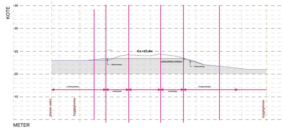
1:500 Profil C
