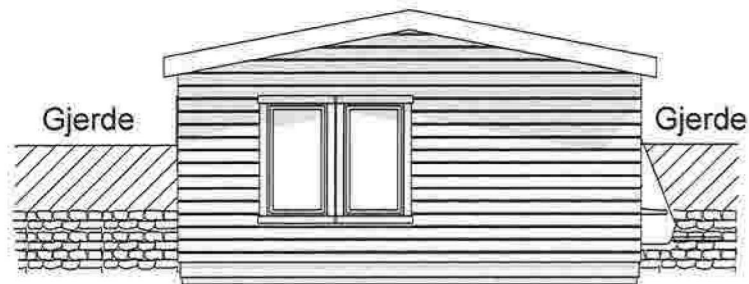
1:100 Fasade Vest
