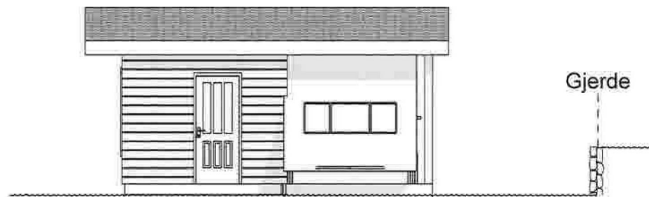
1:100 Fasade Sør
