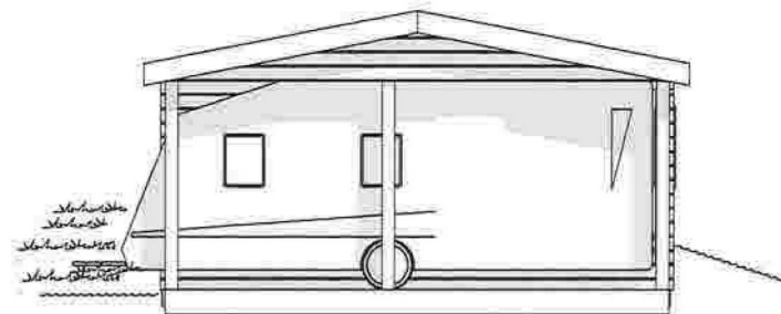
1:100 Fasade Øst
