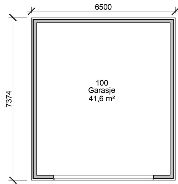
Plan 1 1 : 100
