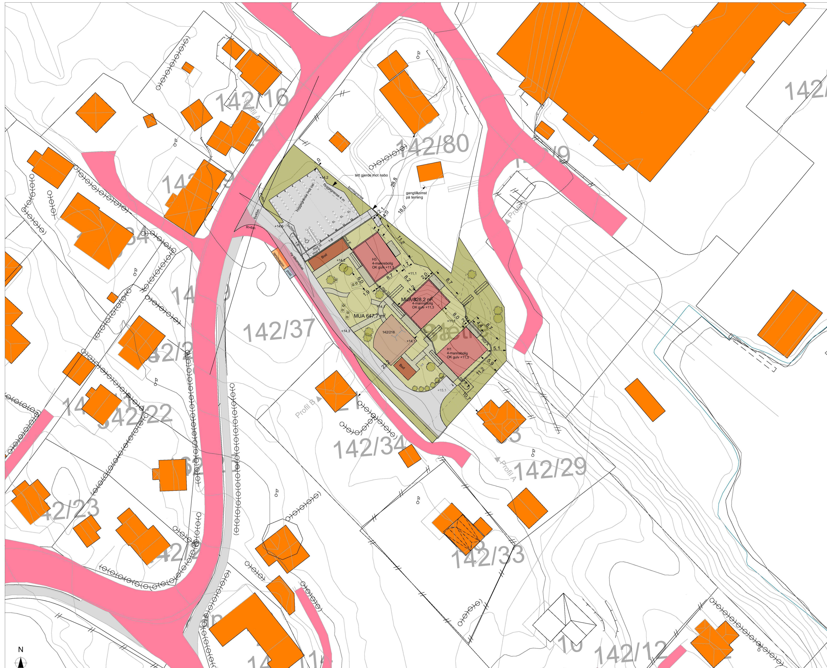
1:500 Situasjonsplan
