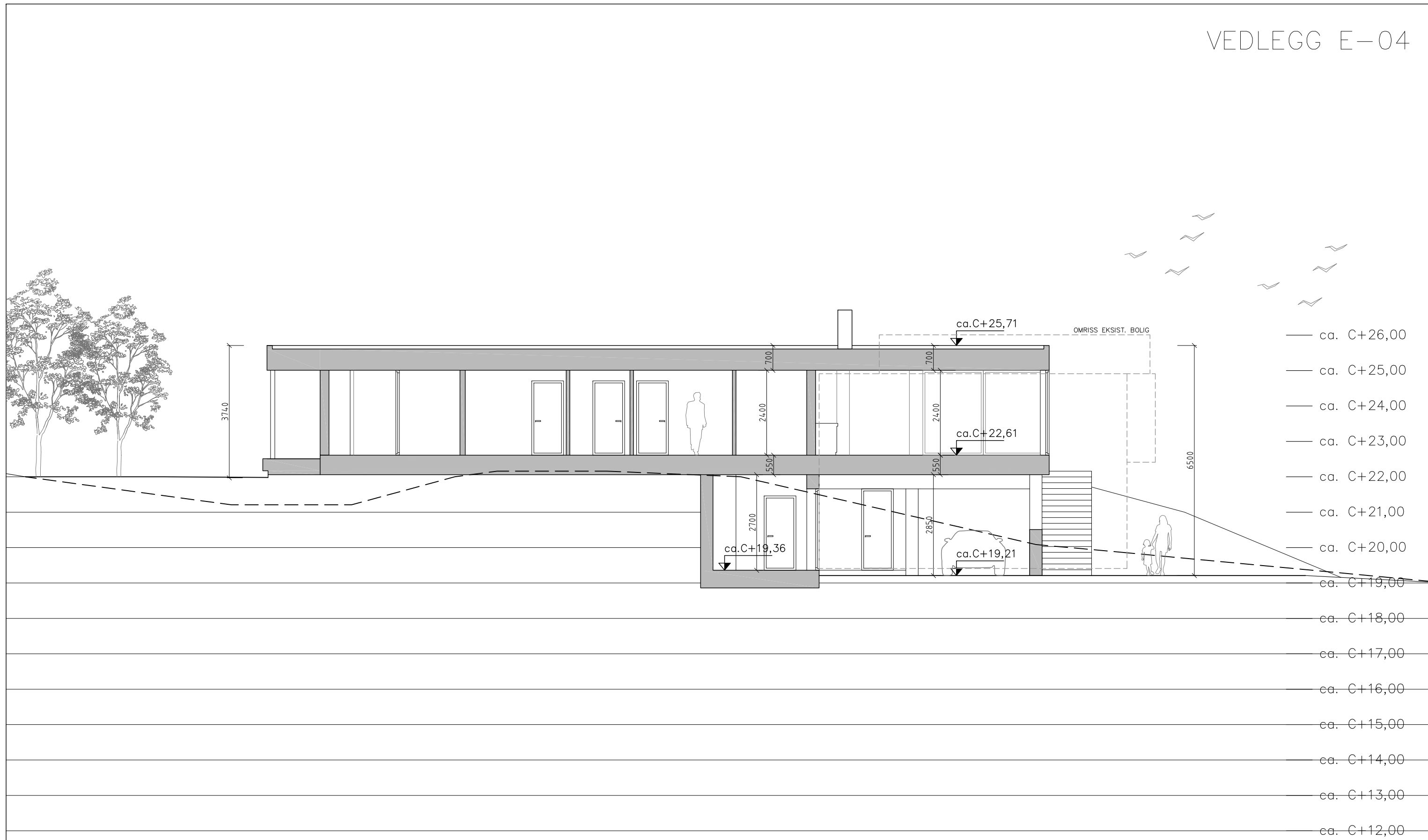
PRINSIPP SNITT A-A NY SITUASJON
