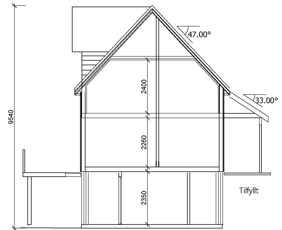
Snitt A
