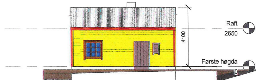
3 Austfasade
