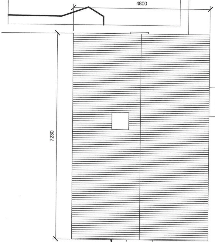
1 Plan tomt 1 : 50
