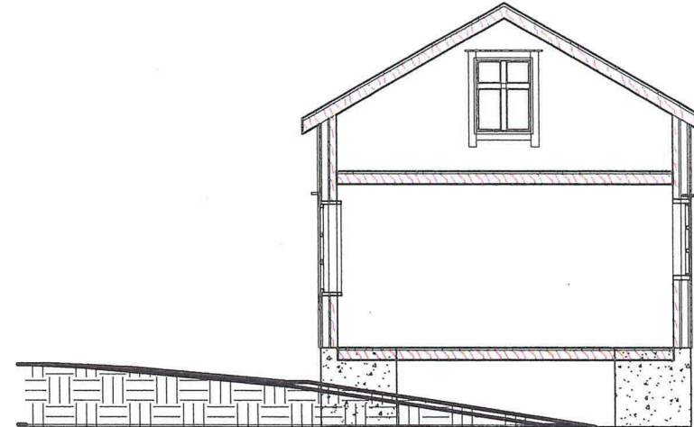
1 Tverrsnitt
