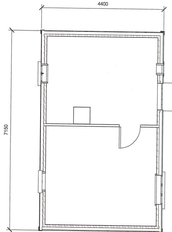
2 Plan 1 etg 1 : 50
