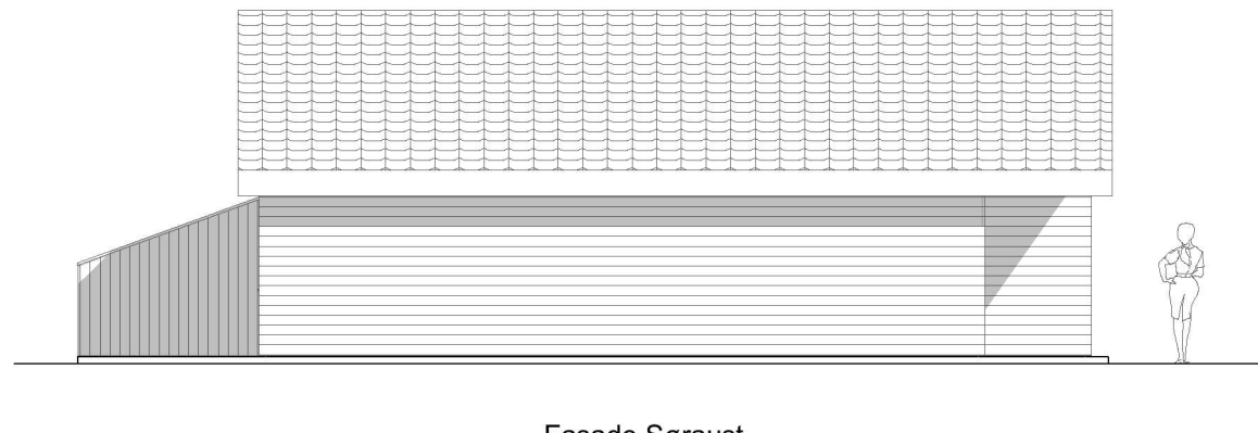
Fasade Søraust
