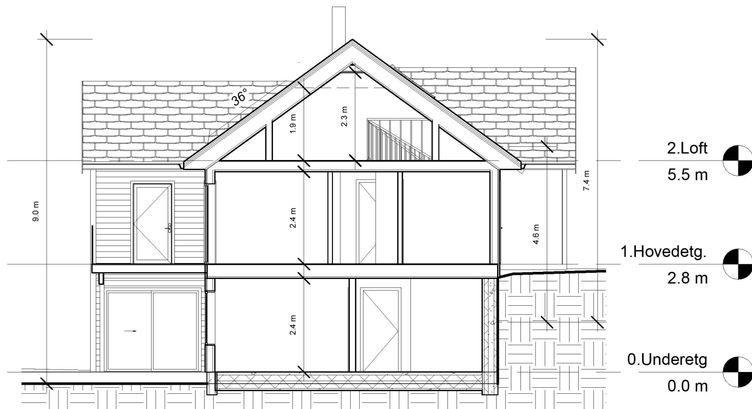
1 Snitt 3 1 : 100
