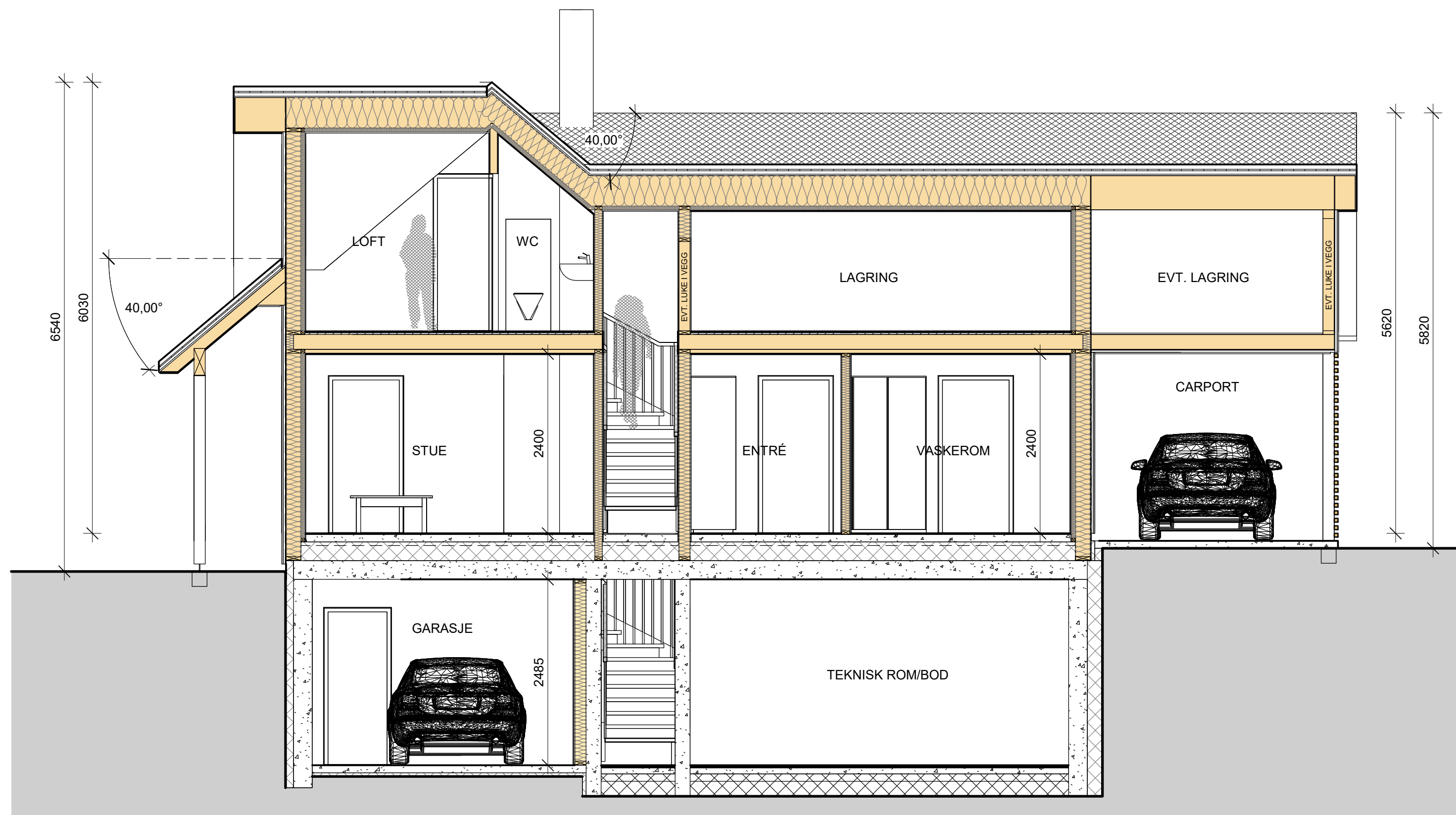
1 Snitt 1 1:50
