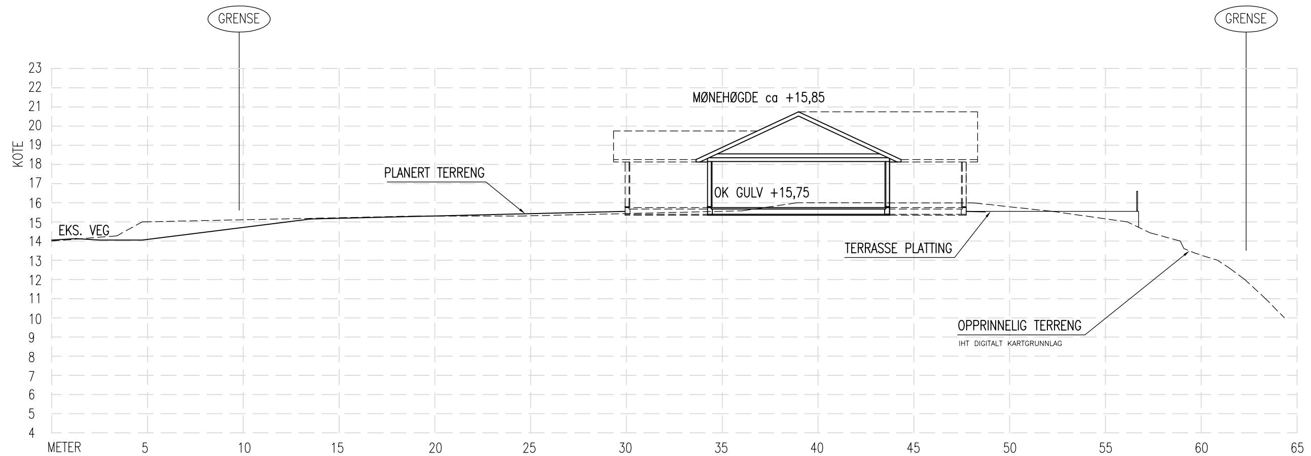
TERRENGPROFIL A-A
