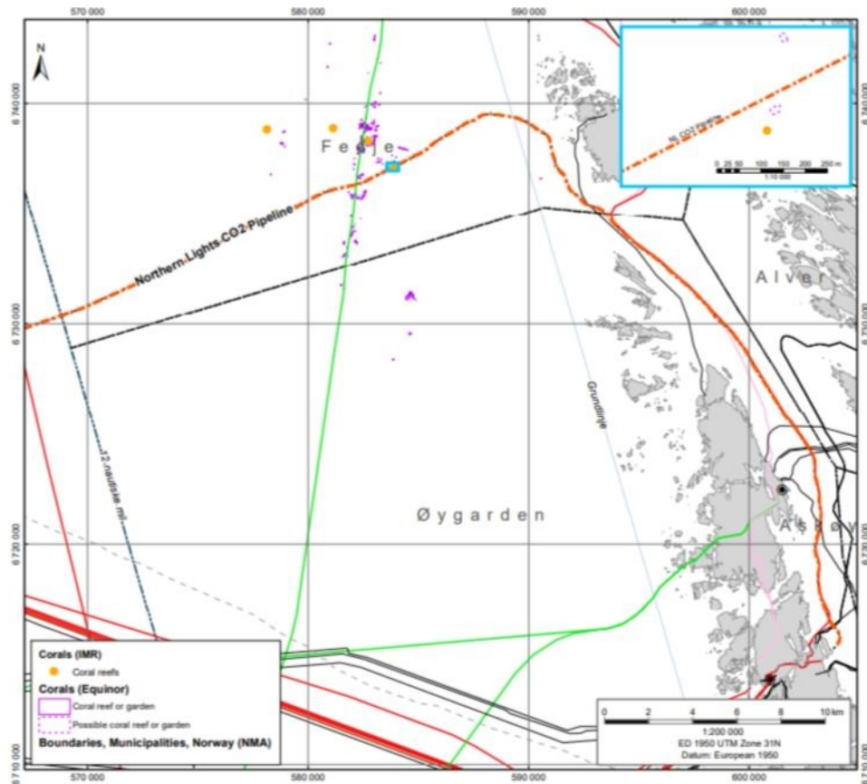
Figur 4. Rørledningstrase og korall-lokasjon.
