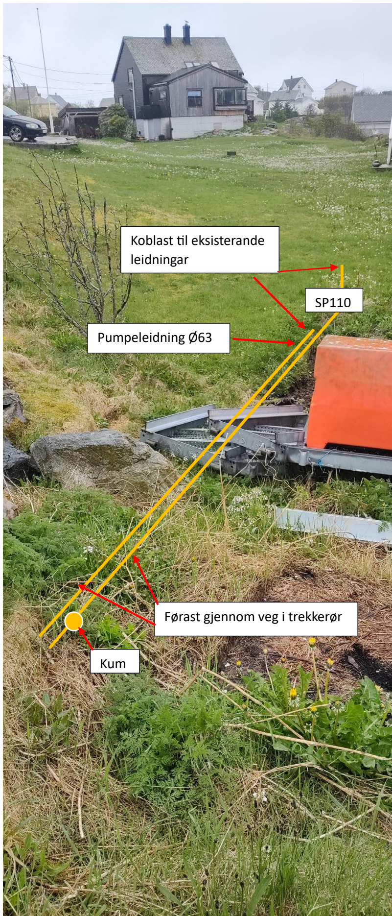
Prinsippskisse til APS frå eksisterande rør
