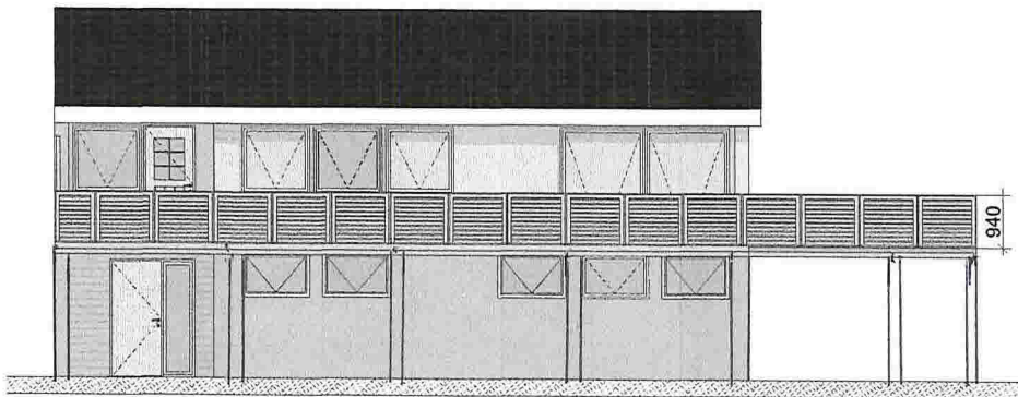
Fasade Sør
