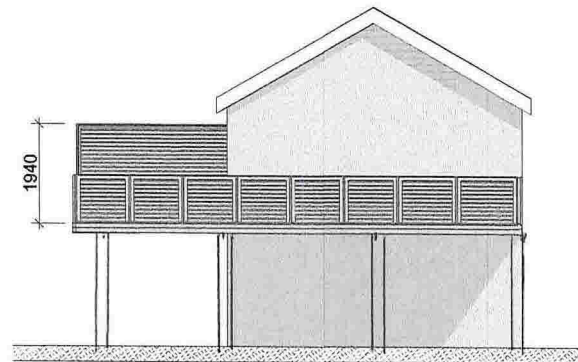
Fasade Øst
