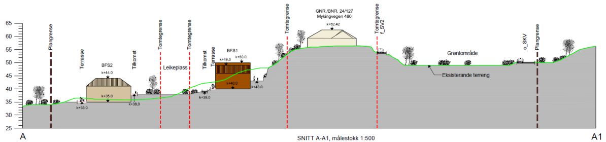
Figur 16: Snitt A-A1
