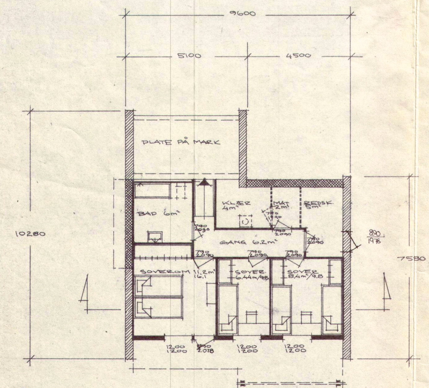
PLAN UNDERETASJE. GRUNNMURTEGNING NR 432409 SANITÆRTEGNING NR. 216002
