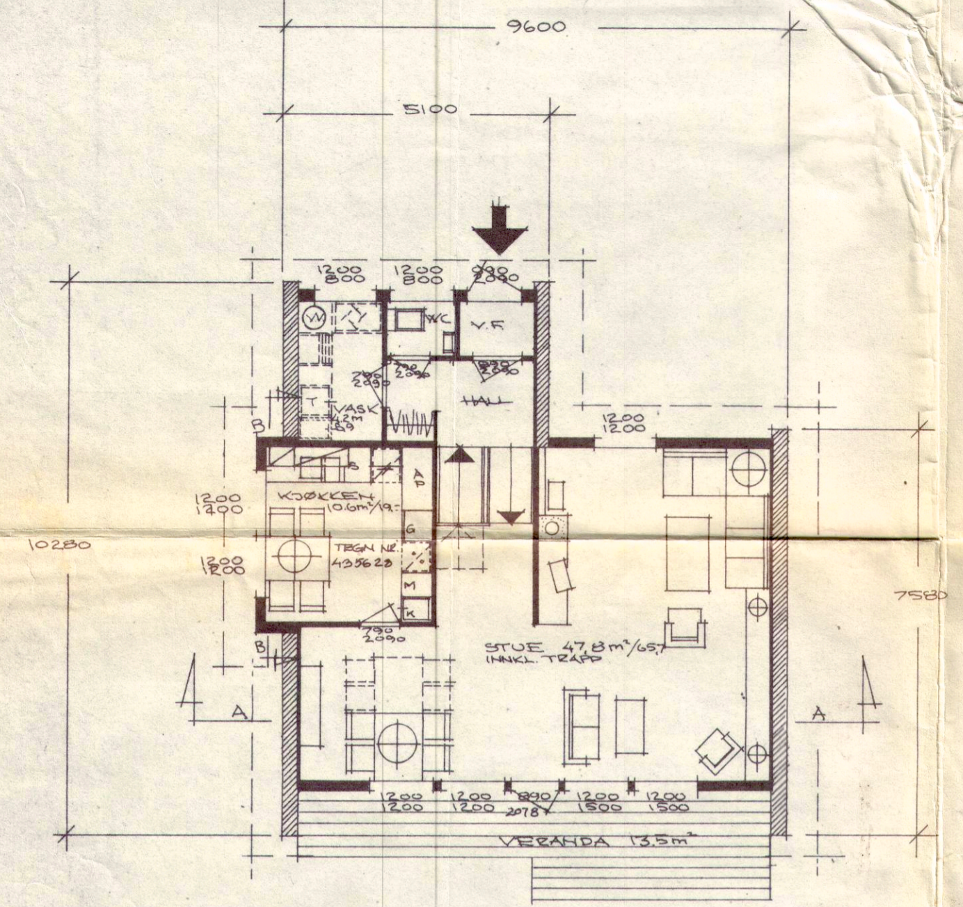
PLAN 1. ETASJE
