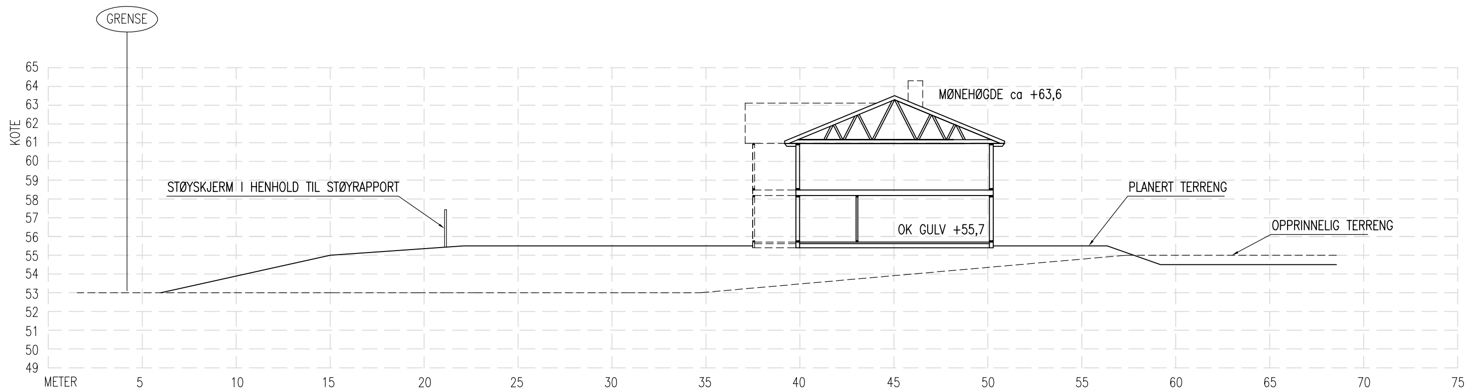
TERRENGPROFIL D-D
