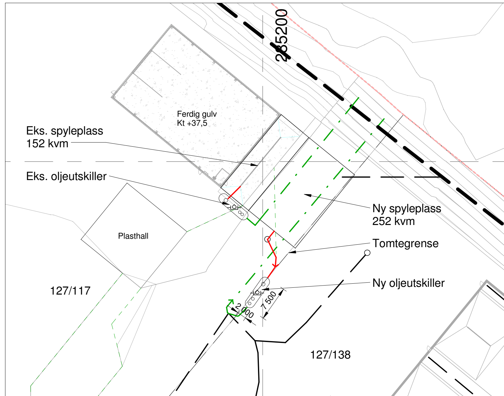
Bunnledningsplan - Spyleplass 1 : 500
