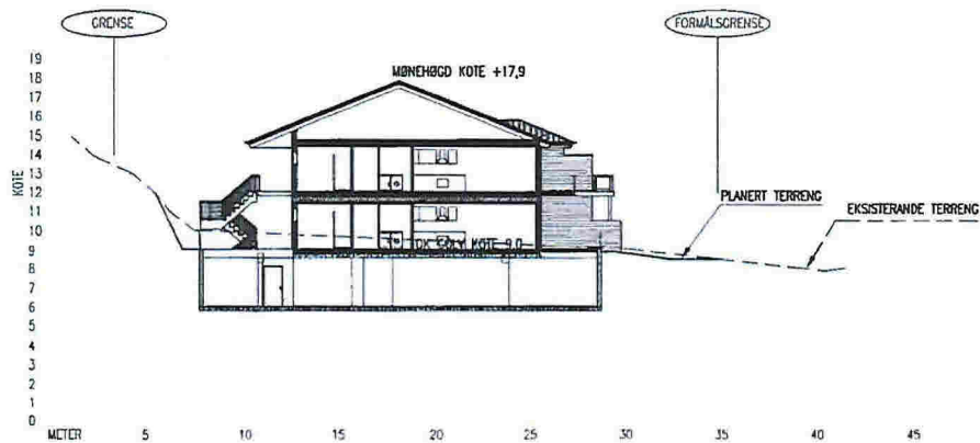
TERRENGPROFIL A-A
