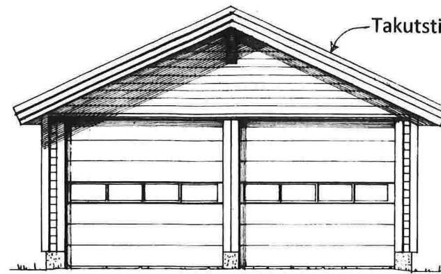
Fasade mot SØR-ØST
