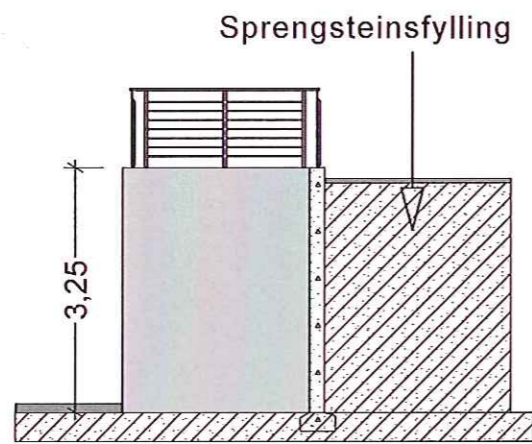
AA snitt 1:100
