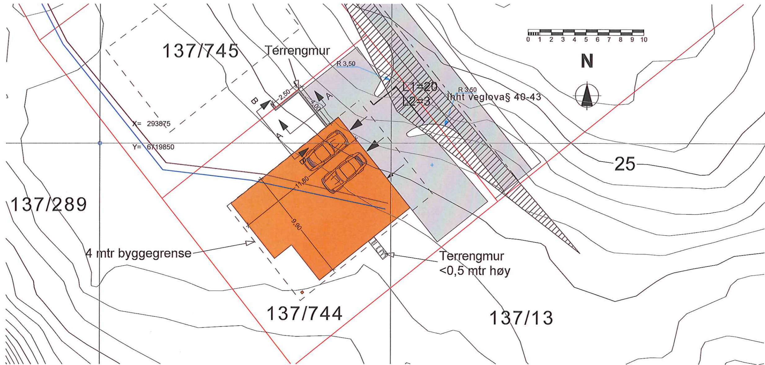
Situasjonsplan terrengmurer 1:200
