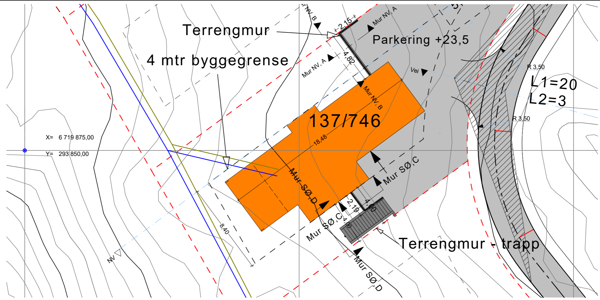
Situasjonsplan terrengmurer 1:200
