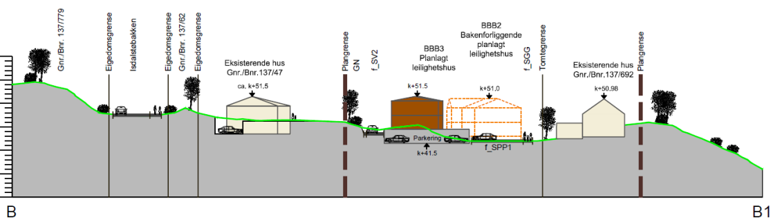
Figur 16: Illustrasjon med snitt for planområdet.
