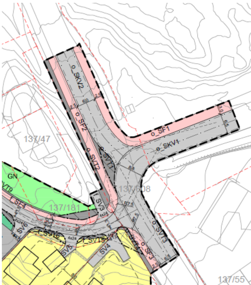
Figur 14: Ny løysing som syner oppdatering av eksisterande kryss til planområdet, samt kryss like nord for dette.
