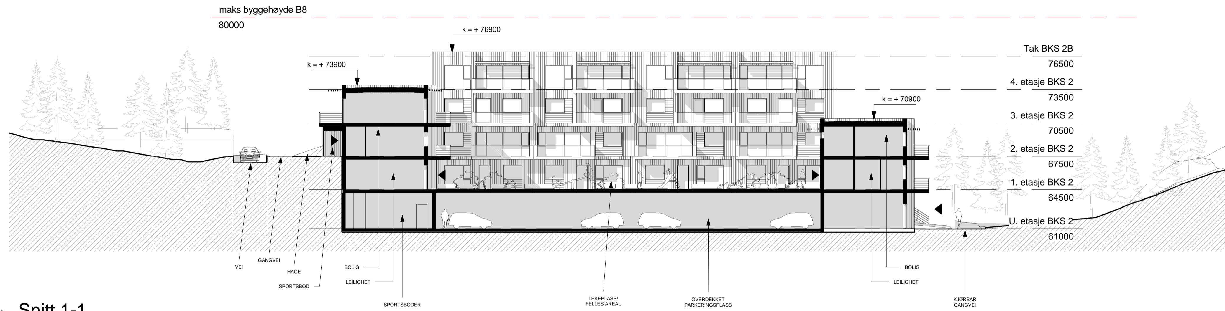
1 Snitt 1-1 1 : 200
