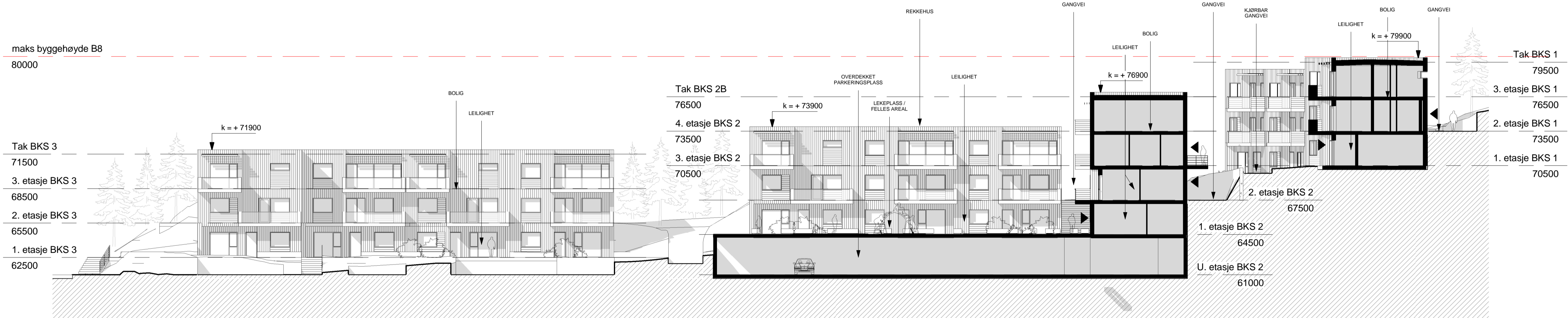
2 Snitt 2-2 1 : 200
