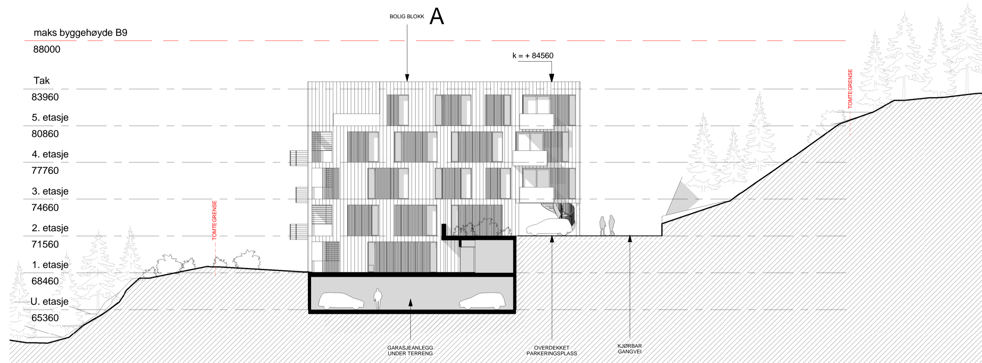
1 3-3 1 : 200
