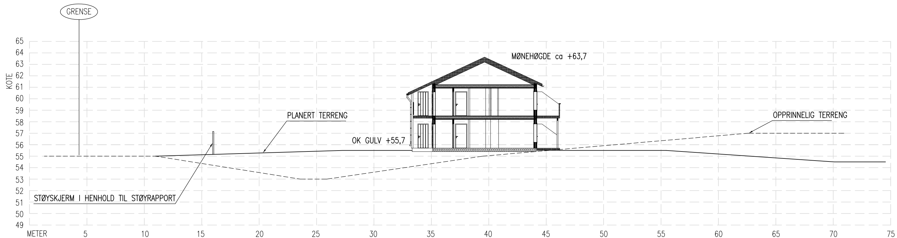
TERRENGPROFIL E-E
