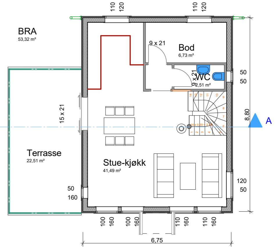
2 etasje 1:100
