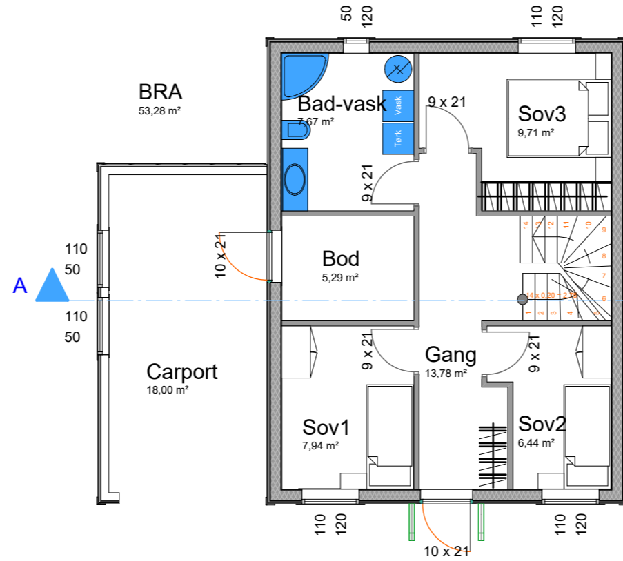
1 etasje 1:100 1.
