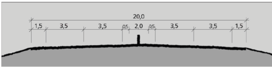
H8: Nasjonale hovudveger og andre hovudveger, ÅDT 12000- 20.000 og fartsgrense 110 km/t if. NA-rundskriv 2015/2 – Fartsgrenser og motorveger – Ny dimensjoneringsklasse for motorveg med fartsgrense 110 km/t. I følge vegnormalen Håndbok N100 er det krav om planskilte kryssningar for standard H8.
