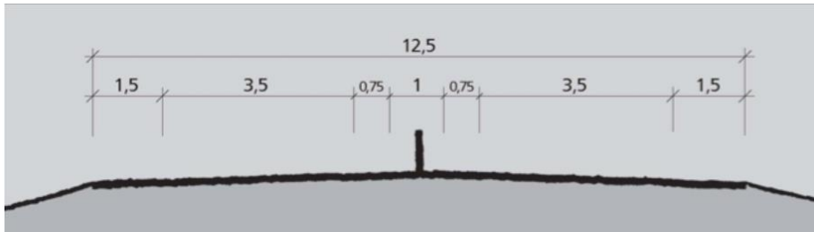
H5: Nasjonale hovudveger og andre hovudveger, ÅDT 6000-12000 og fartsgrense 90 km/t. I følge Vegnormalen Håndbok N100 er det krav om planskilte kryssningar for standard H5 ved ÅDT over 8000.
