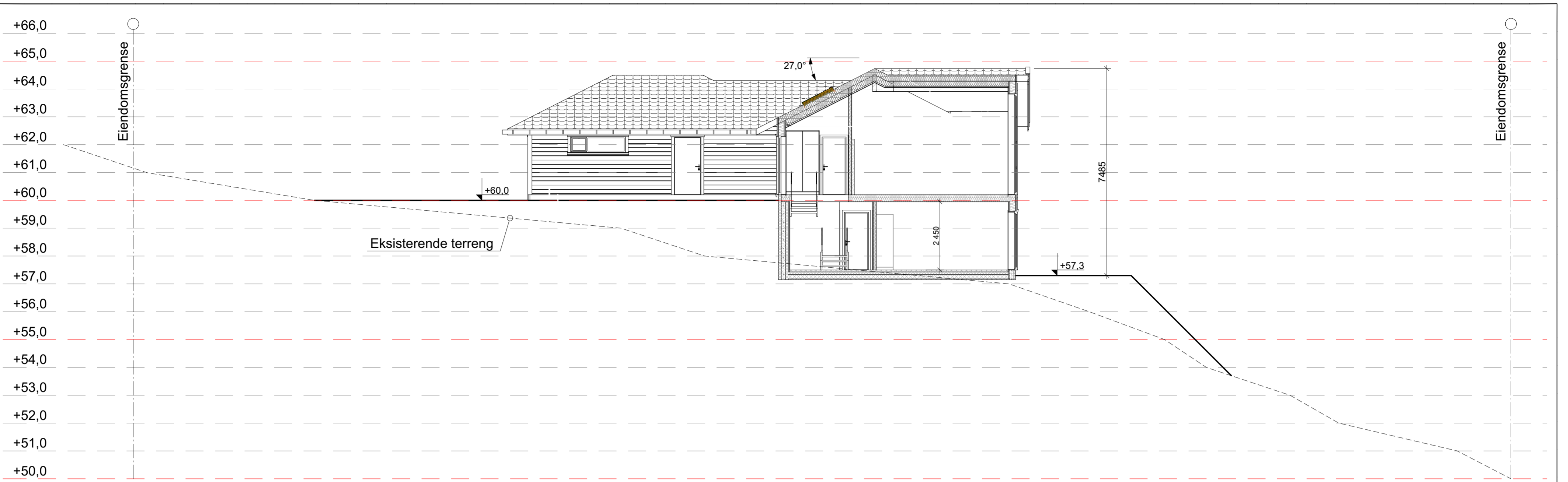
snitt A - A
