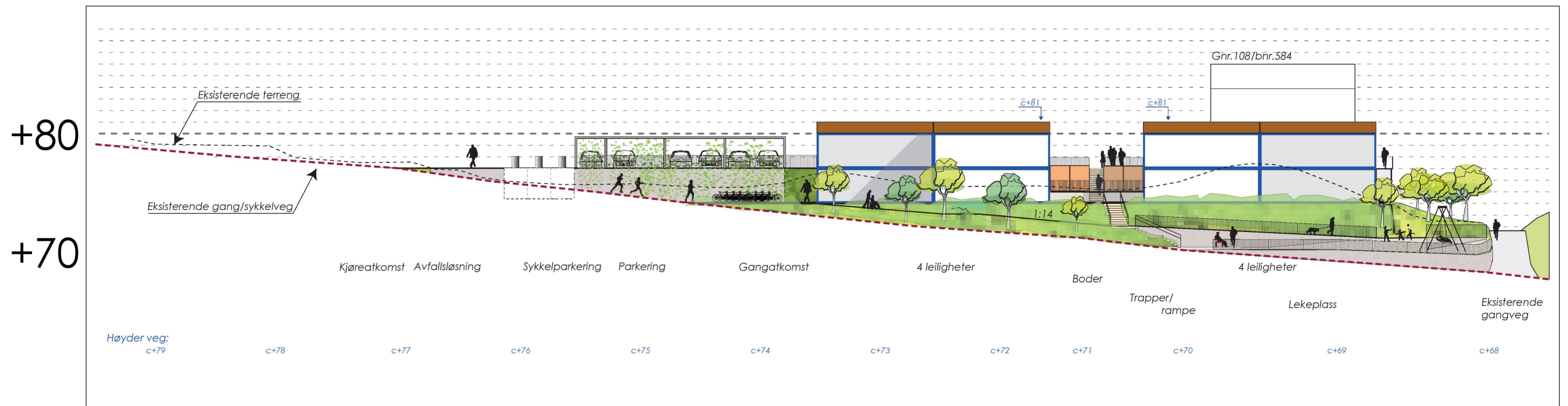
SNITT/OPPRISS Aa
