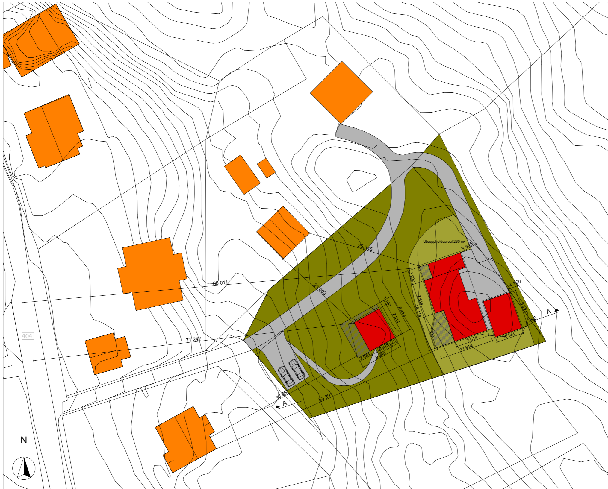
1:500 Situasjonsplan
