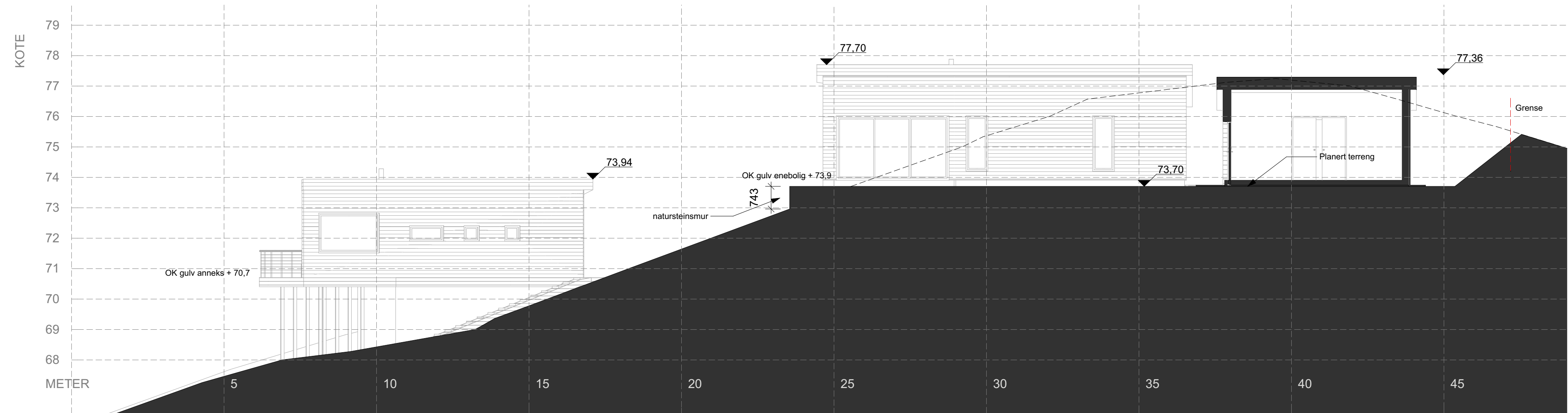
1:100 Terrangprofil A
