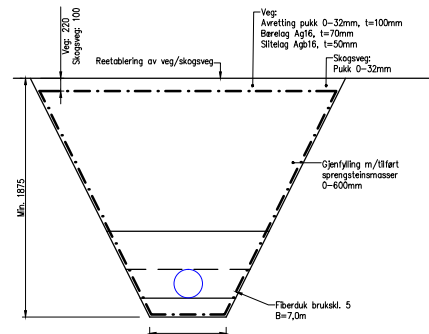
GRØFTESNITT 2. M=1:20 Vannledning i veg/skogsveg
