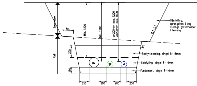
TYPISK GRØFTESNITT. M=1:20 Vann-, spillvann- og overvannsledning
