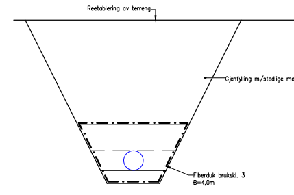
GRØFTESNITT 3. M=1:20 Vannledning i terreng
