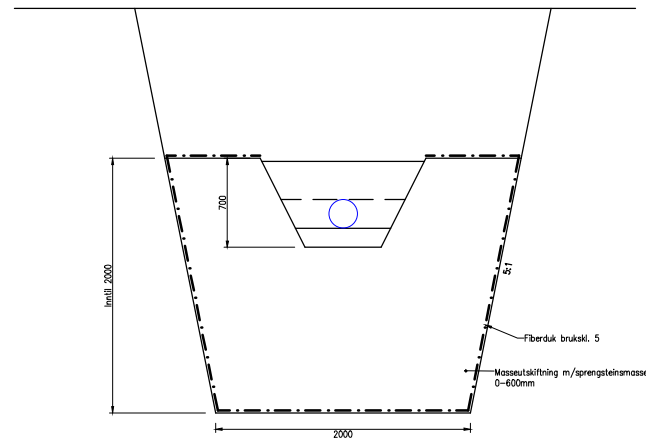
GRØFTESNITT 4. M=1:20 Masseutskiftning for ledningsgrøft
