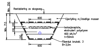
GRØFTESNITT 1. M=1:20 Vannledning i grunn, isolert grøft
